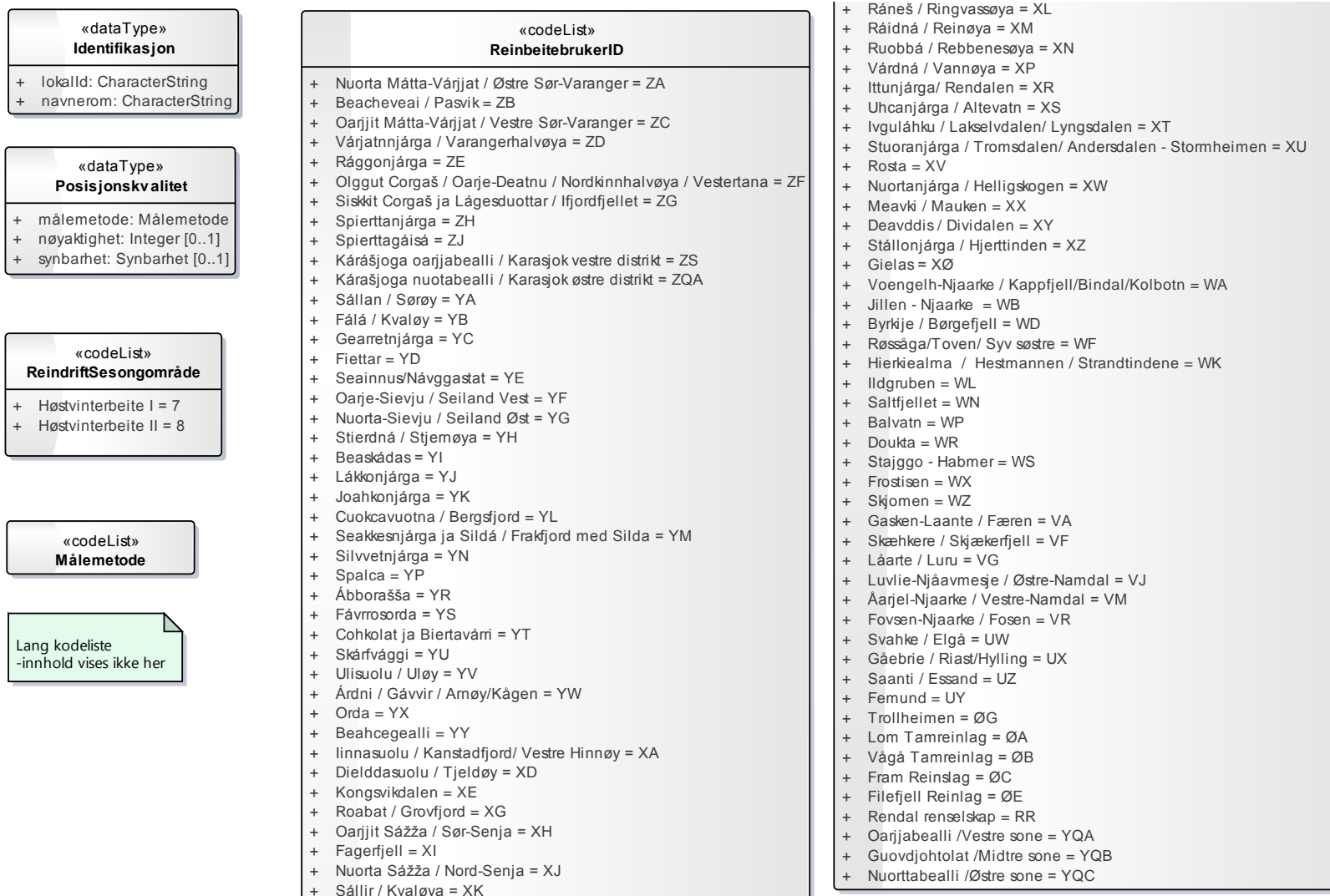
Figur 5 Datatyper og kodelister
